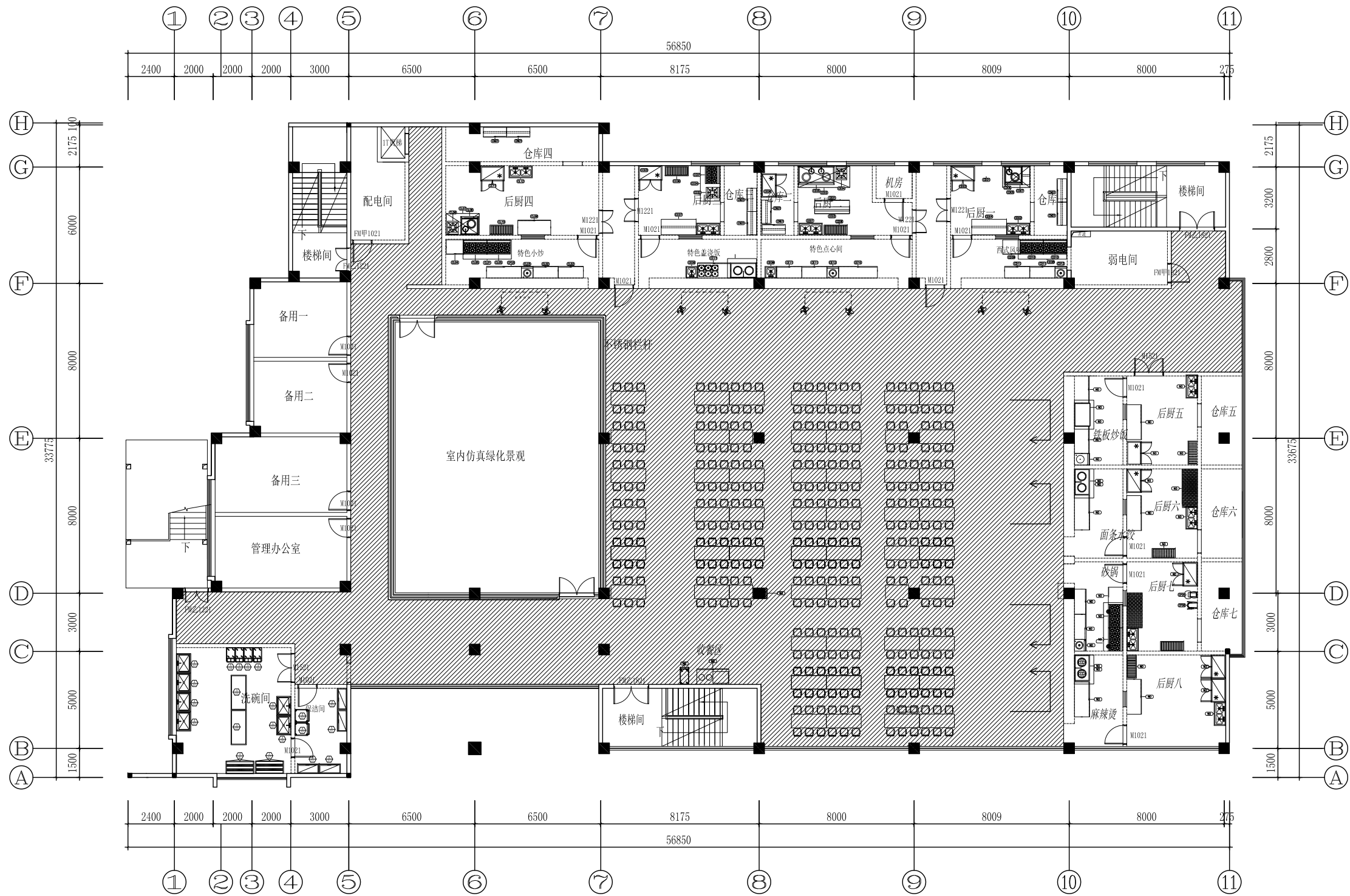
P1 三层平面布置图 3F PLAN 比例: 1:175
